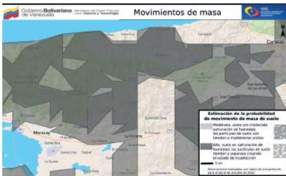
Mapa de movimientos de masa. Región central, estado Aragua
