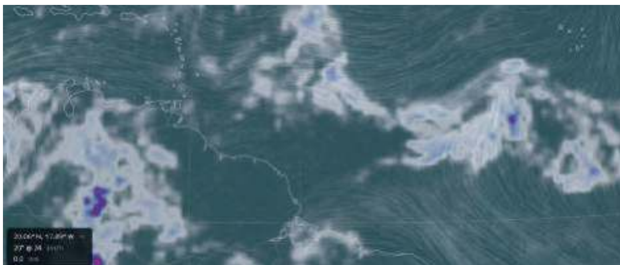
Imagen de centros de baja presión atmosférica en el océano Atlántico movilizándose hacia el mar Caribe el 14 de octubre de 2022
