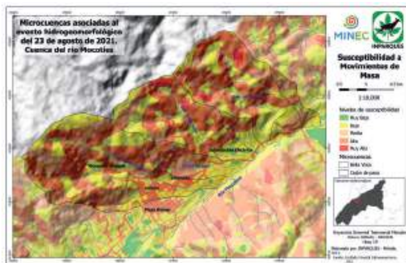
Mapa de susceptibilidad a movimientos de masa. Tovar, Mérida
