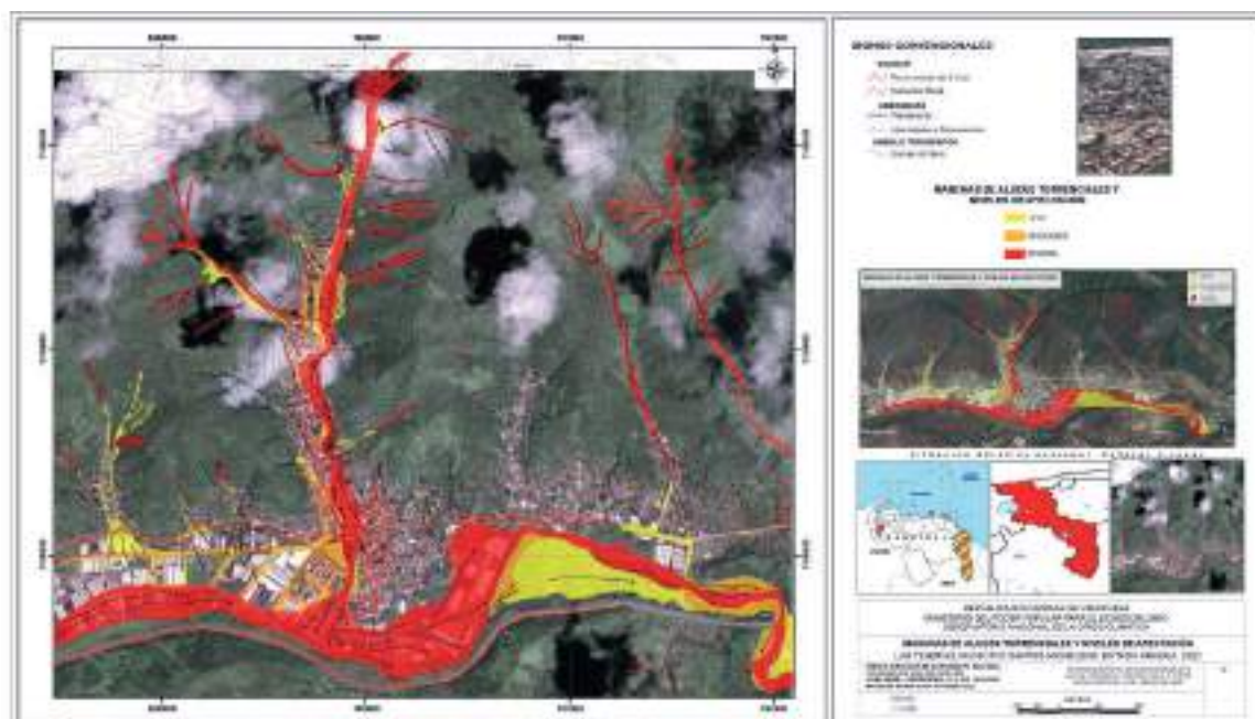
Mapa de mancha de aludes torrenciales y niveles de afectación. Las Tejerías, Aragón
